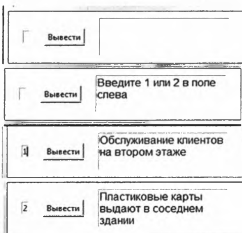
Рис. 5.24. Графический интерфейс
